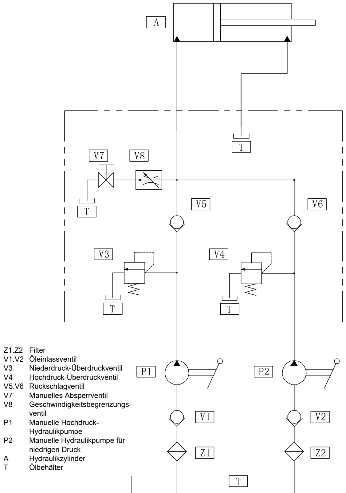
Abb. 11: Hydraulikplan
