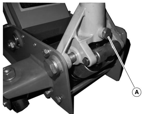
Abb. 5: Feststellschraube
