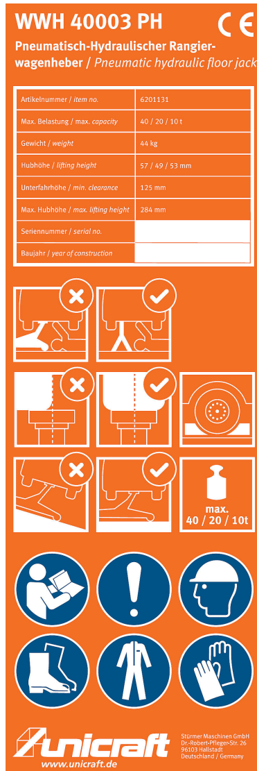
Abb. 1: Sicherheitskennzeichnung und Typenschild WWH 40003 PH
